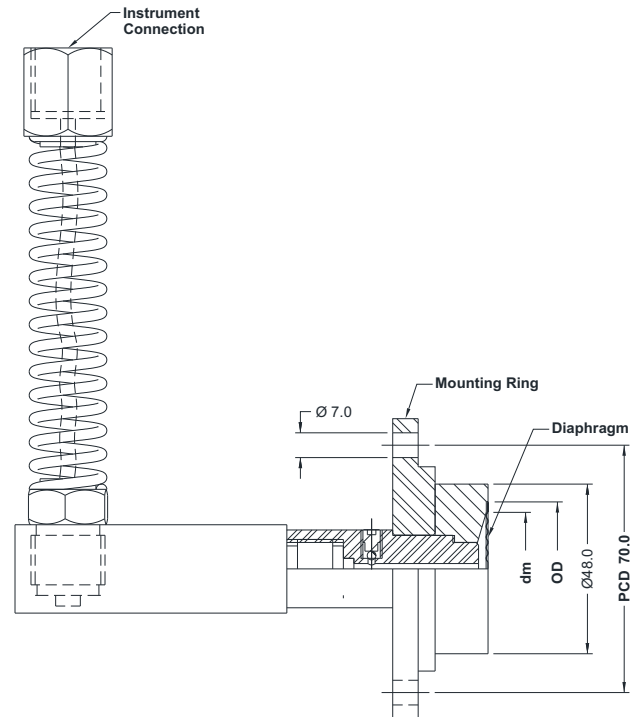
ASSEMBLY : B5
